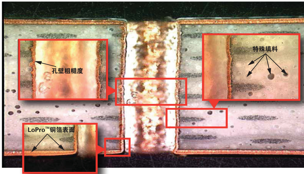
图1: RO4700板材镀铜孔后的切片图。需要注意的是这种特别填料会稍微增加孔壁的粗糙度,对于这种板材是正常的。另外LoPro铜箔在表面涂了一层薄的改性的无色树脂。建议第一次加工RO4700板材之前请与Rogers公司的技术支持工程师讨论孔壁品质和外观现象。
